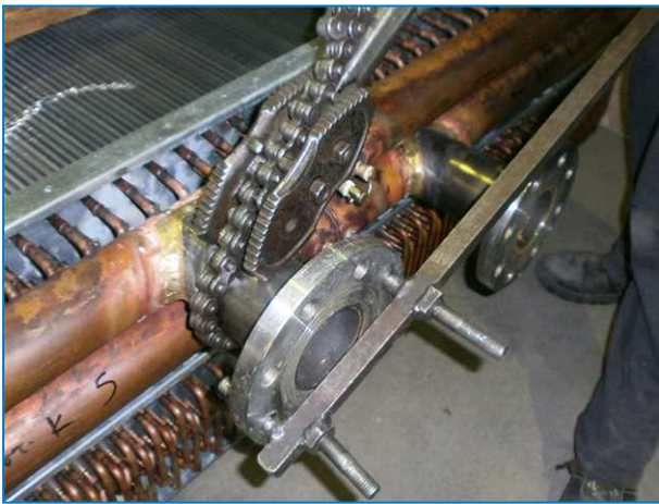
Installazione flangia avvitabile
