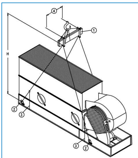
Метод монтажа изделий HFL
