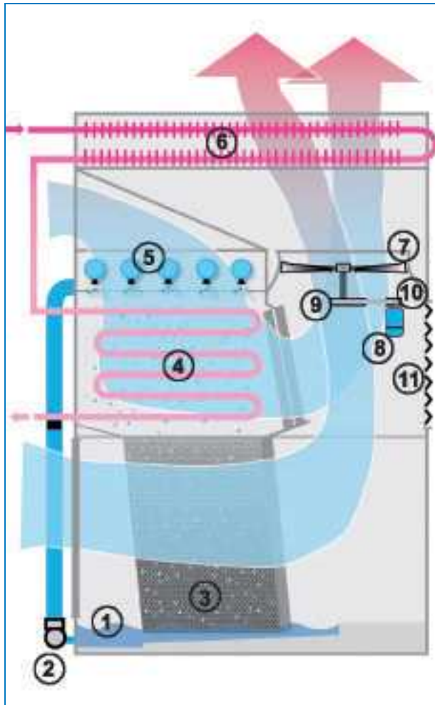
Principio di funzionamento - Ammortizzatori di Ingresso Aria modulanti chiusi.
