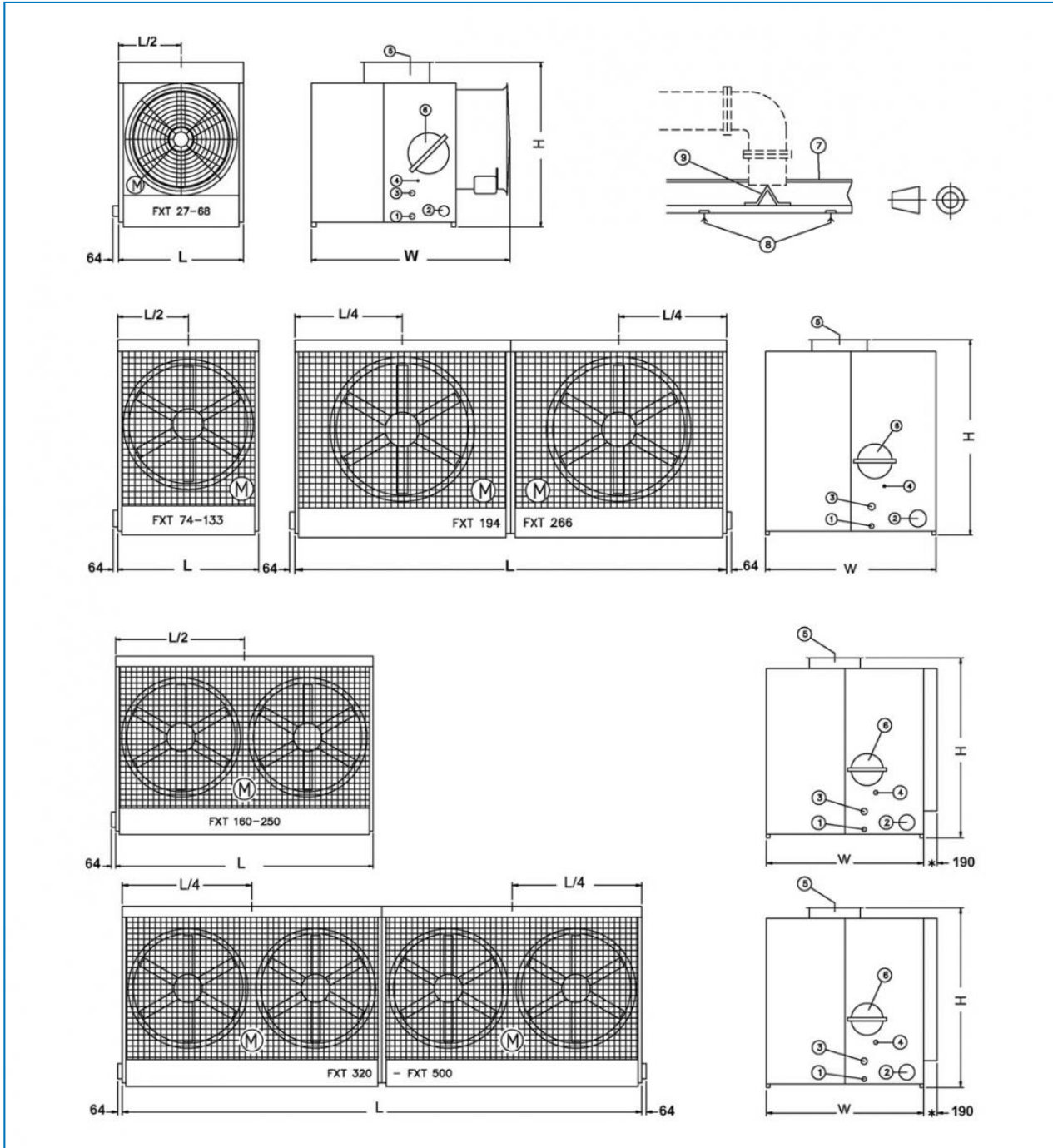
1. Drenaggio; 2. Uscita acqua; 3. Troppopieno; 4. Reintegro; 5. Entrata acqua; 6. Portello d'ispezione; 7. Sommità vasca di distribuzione; 8. Ugelli calibrati; 9. Separatore del flusso; * Sezione reti esterne solo su FXT 211, 250, 422, 500.
