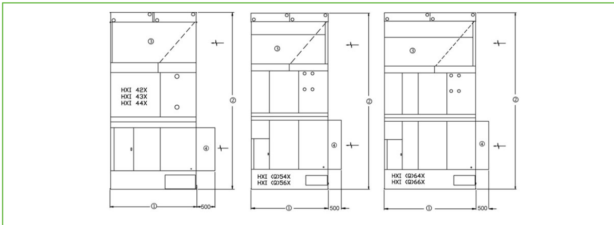
1. Larghezza unità; 2. Altezza unità; 3. Plenum coibentato; 4. Attenuatore in aspirazione.
