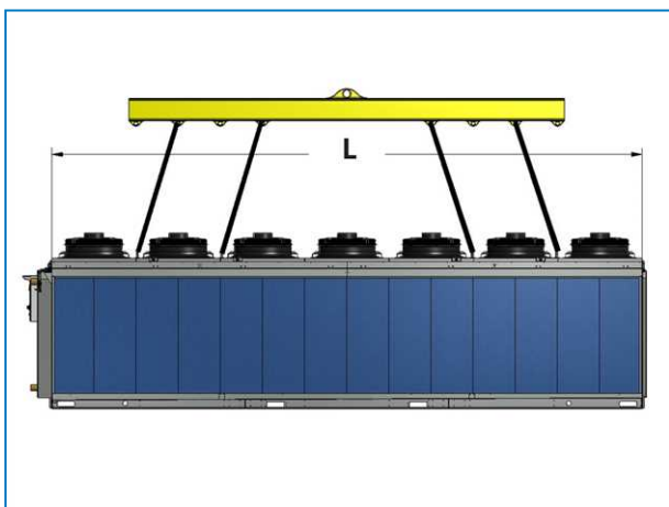
Изделия с 14 вентиляторами
