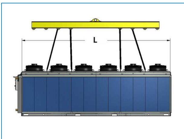
Изделия с 12 вентиляторами
